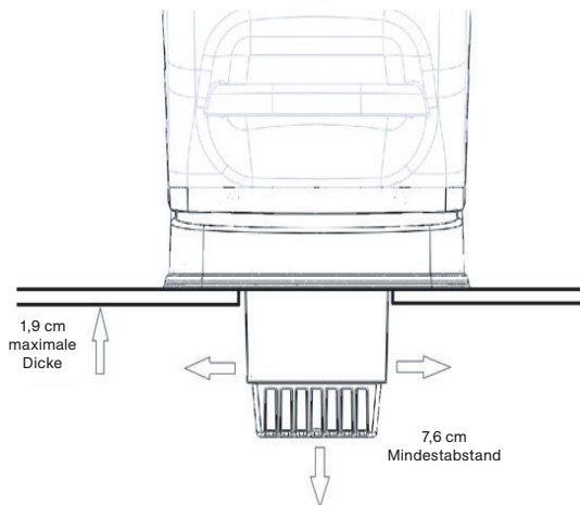
Abbildung 3. Stealth-Einbau in die Theke - Abstand
