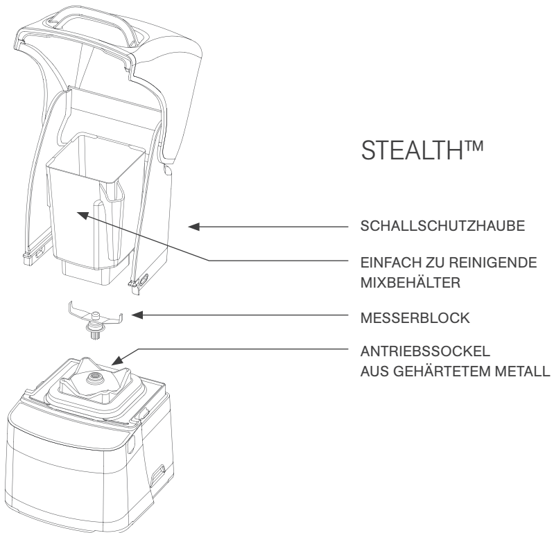
Abbildung 2. Stealth-Komponenten
